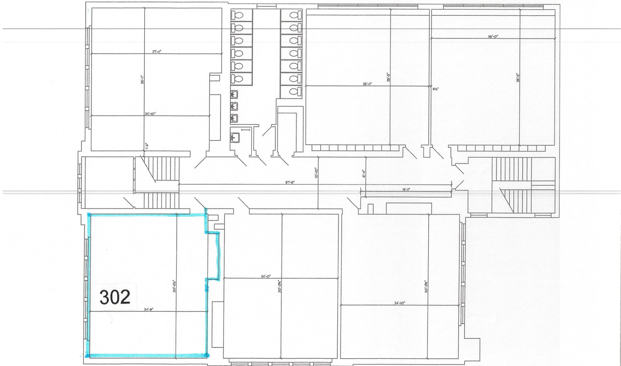
SCALE: 3/32" = 1'-0"
