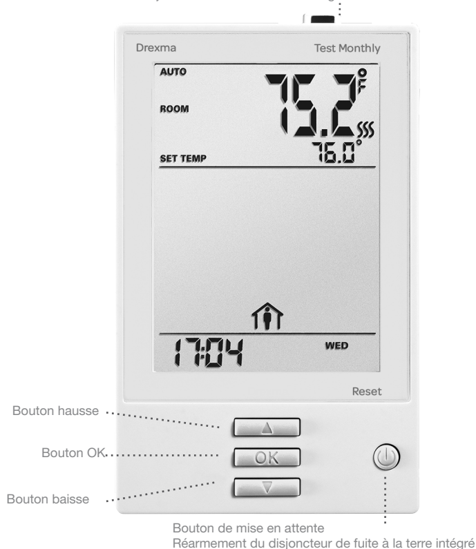
Bouton d'essai du disjoncteur de fuite à la terre intégré
