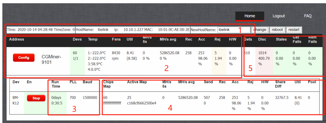
图 5 eLink K1 矿机网页主页
