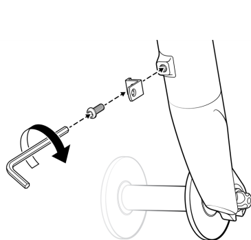
Installation du support en L (nécessaire sur certains vélos)
