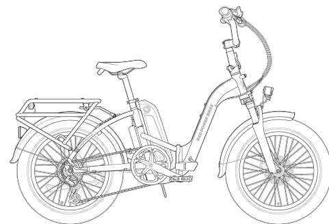
Assemblage complet du RadExpand 5 Plus
