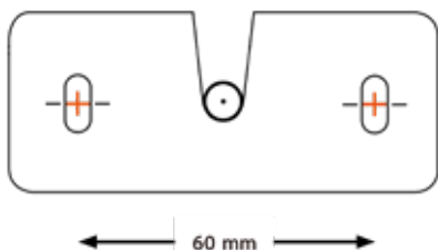
Abb. 03: Bohrlöcher
