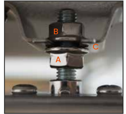
Abb. 07: Wandmontage
