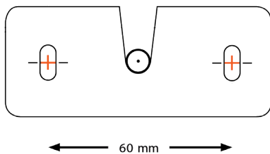
Abb. 03: Bohrlöcher
