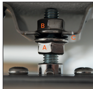
Abb. 07: Wandmontage
