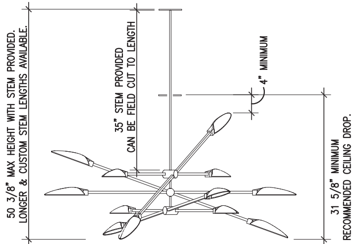
ELEVATION
