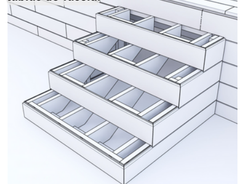
Fije clips para tablas de borde y tablas ranuradas y fije las tablas en su sitio.
