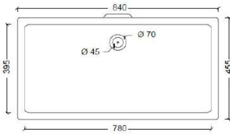
CORNELIA 845 × 460 × 155 MM
