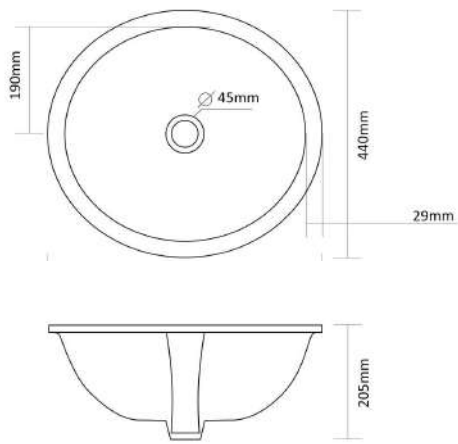
SELENE 490 × 440 × 205 MM
