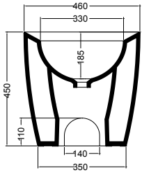
SEZIONE LONGITUDINALE LONGITUDINAL VIEW
