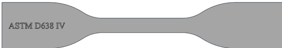
Figure 1 Tensile bar
