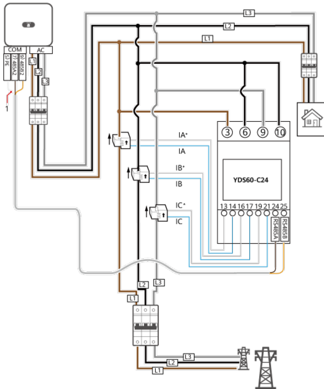
Abbildung 5-24 Dreiphasige, dreiadrige Kabelverbindung mit YDS60-C24 (Smart Dongle- Vernetzung)
