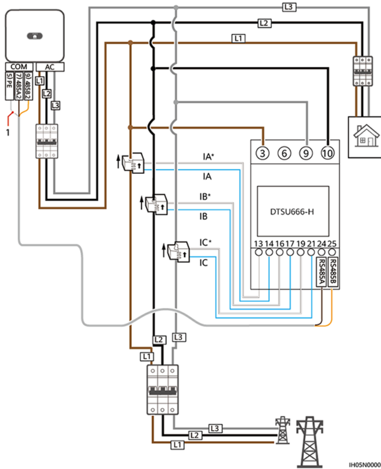
Abbildung 5-23 Dreiphasige, dreiadrige Kabelverbindung mit DTSU666-H (Smart Dongle- Vernetzung)
