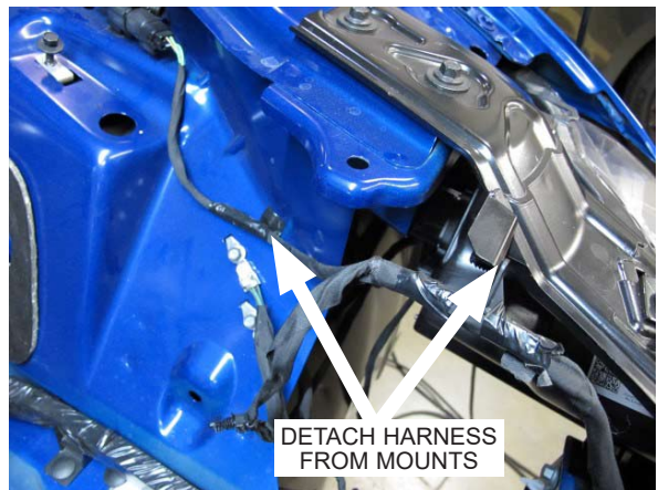
Fig. 4-al: Detach Harness
