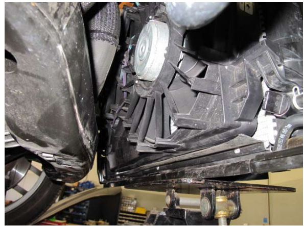
Fig. 2-t: Remove radiator fan assembly
