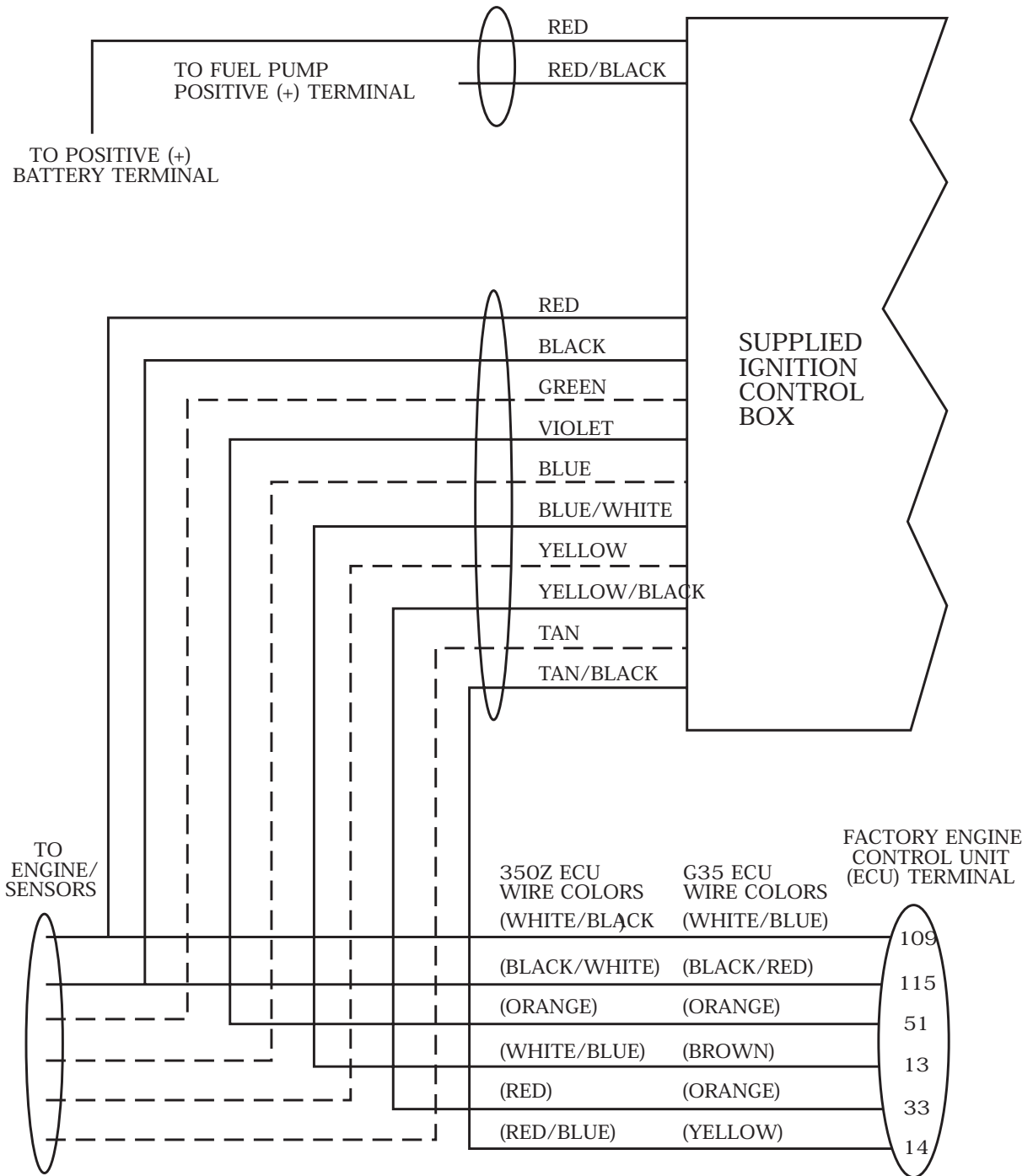
Fig. 10-d / Wiring Diagram
