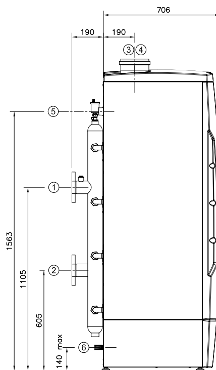
VISTA LATERAL
