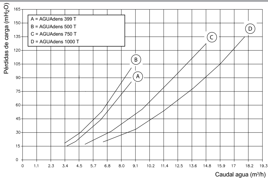
PÉRDIDAS DE CARGA AGUAdens T
