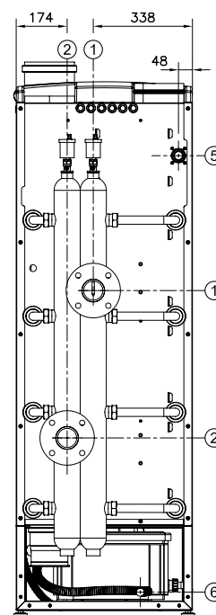
VISTA TRASERA
