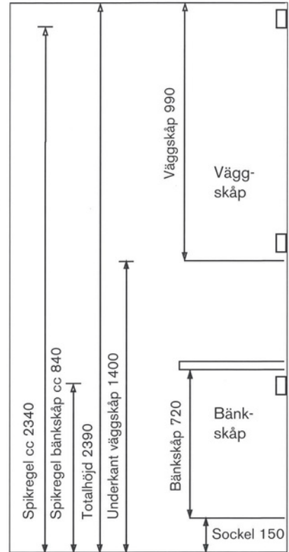
Väggskåp höjd 990 mm
