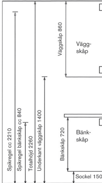
Väggskåp höjd 860 mm
