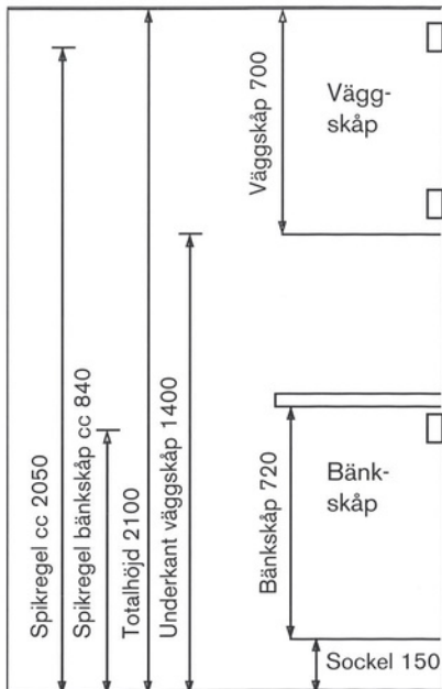
Väggskåp höjd 700 mm
