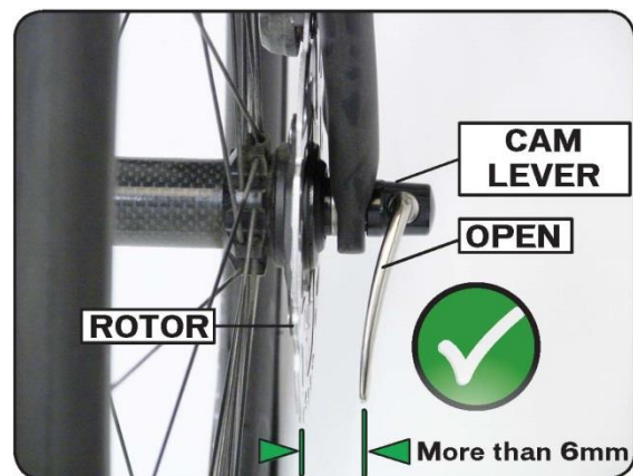
圖2. 快拆杆跟碟盤有足够的間隙
