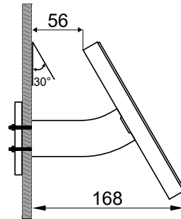
Seitenansicht
