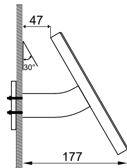
Seitenansicht
