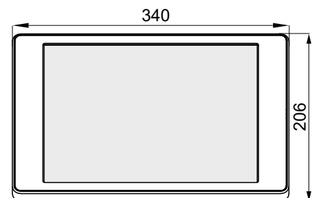
Frontansicht
