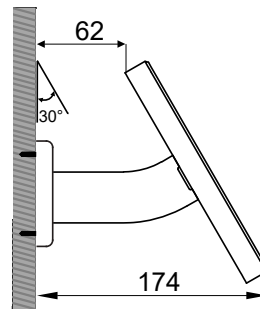
Seitenansicht
