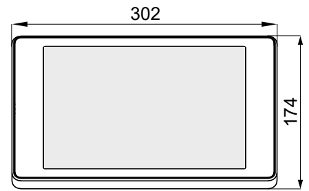
Frontansicht
