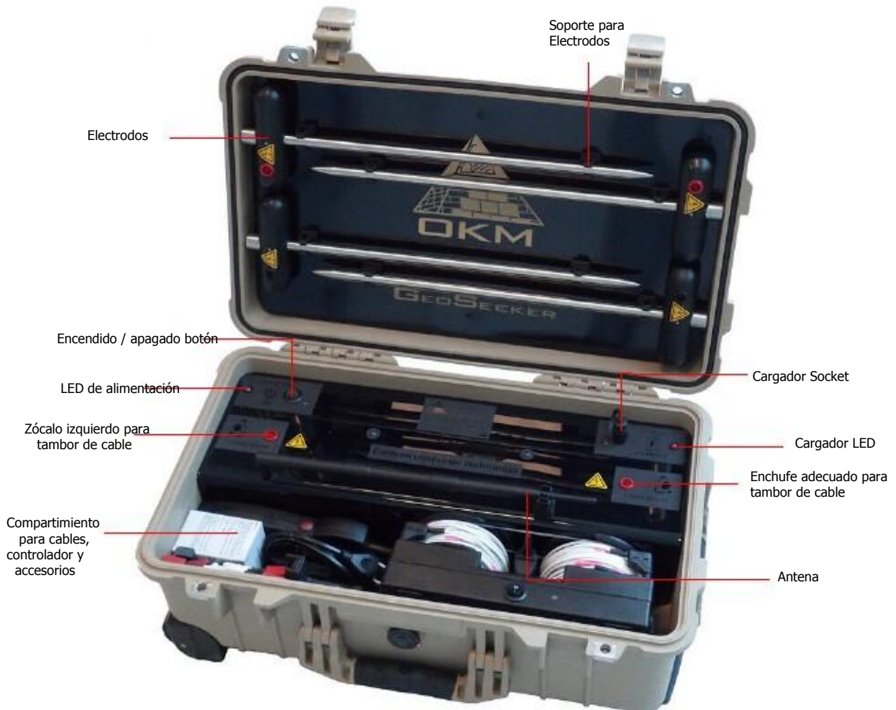
Figura 4.6: Elementos de control de la caja de alimentación
