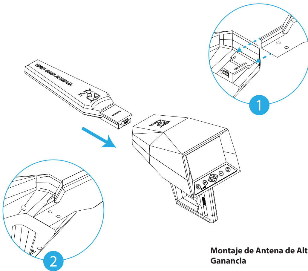
figura 5 -Antena de Alta Ganancia Montaje.
