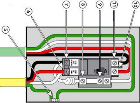
Boîte de disjoncteur GFCI
