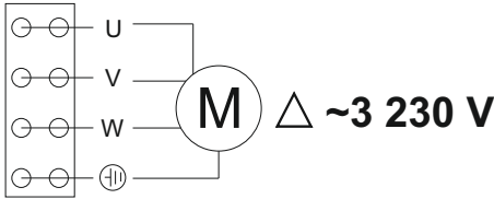
Fig. 6a EN 61800-3 Class C2
