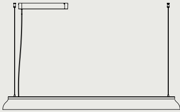
PC Linear Lamp W120 X D14 x H10 cm
