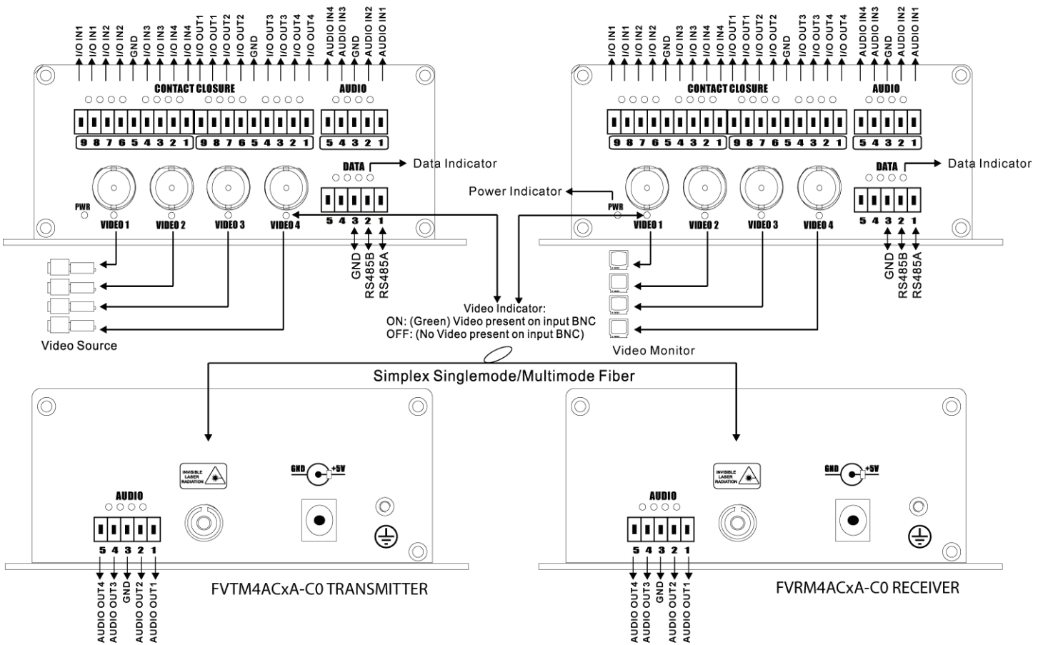
FVTM4ACxA-C0 TRANSMITTER
