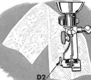
Fig. 52. The Edge Stitcher
