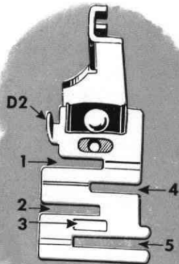
Fig. 52. The Edge Stitcher
