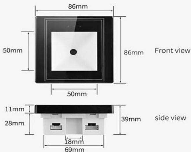
Abmessungen des ID IDENT 1500
