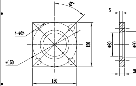
Flange
