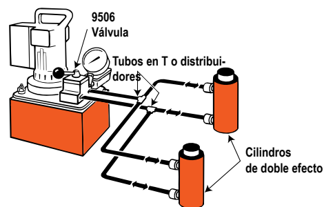
Cilindro o cilindros de doble efecto en el circuito, controlados por una válvula montada en bomba.
