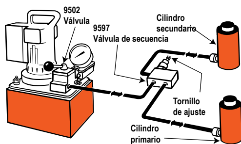
Cilindros de simple efecto con válvula de secuencia que controla los circuitos de los cilindros primario y secundario.
