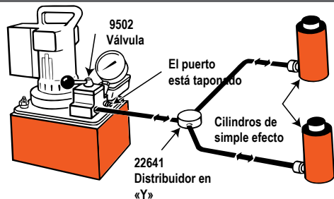
Cilindros de simple efecto o cilindros en el circuito, controlados por una válvula montada en bomba.
