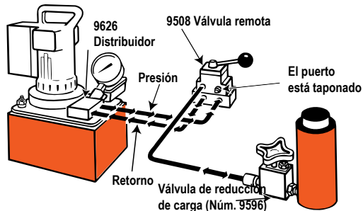
Cilindro de simple efecto controlado por una válvula montada de forma remota.
