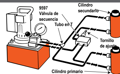
Cilindros de doble efecto con válvula de secuencia que controla los circuitos de los cilindros primario y secundario.
