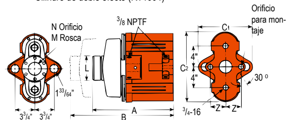
Cilindro de doble efecto (RT1004)
