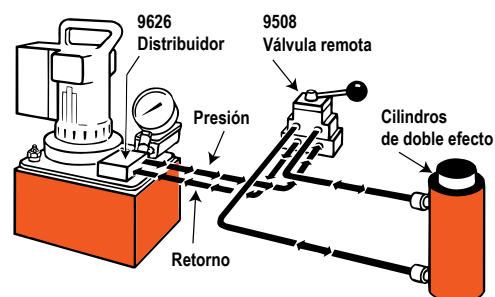
Cilindros de doble efecto controlados por una válvula montada de forma remota.
