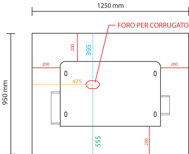
Figura 2 - Schema basamento (misure in mm) Vista dall'alto
