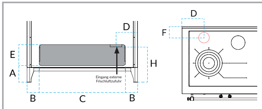
Abb. 12 - Hinteransicht des Sockels und Angaben für den Anschluss an die externe Frischluftzufuhr.
