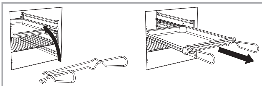
Abb. 16 - Backblechhalter.
