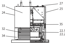
Brennertopf-Ausführung mit Auflage
