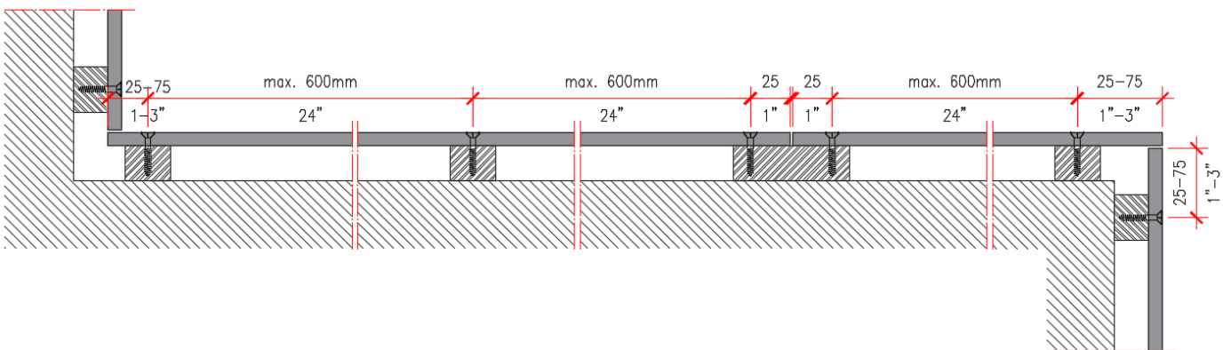
Schéma 2.21 – Coupe horizontale, structure en bois
