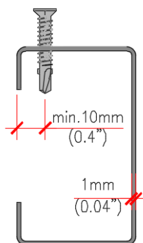
Schéma 2.15 – Distance minimum entre la vis et la limite du profilé métallique
