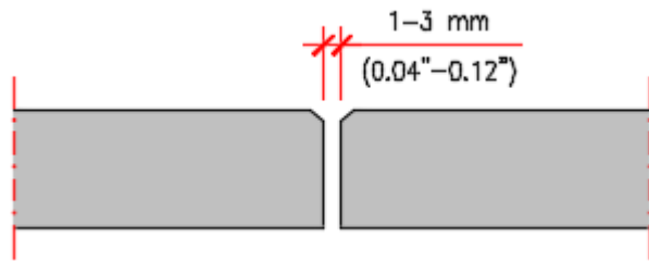
Schéma 3.15 – Arêtes usinées sous forme de biseau
