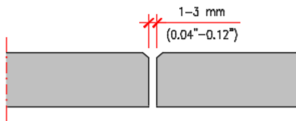
Schéma 2.26 – Arêtes usinées en forme de biseau
