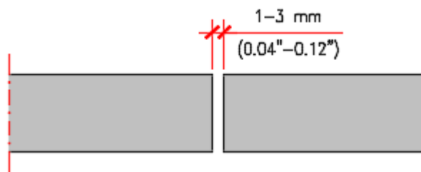
Schéma 3.13 – Joints entre panneaux
