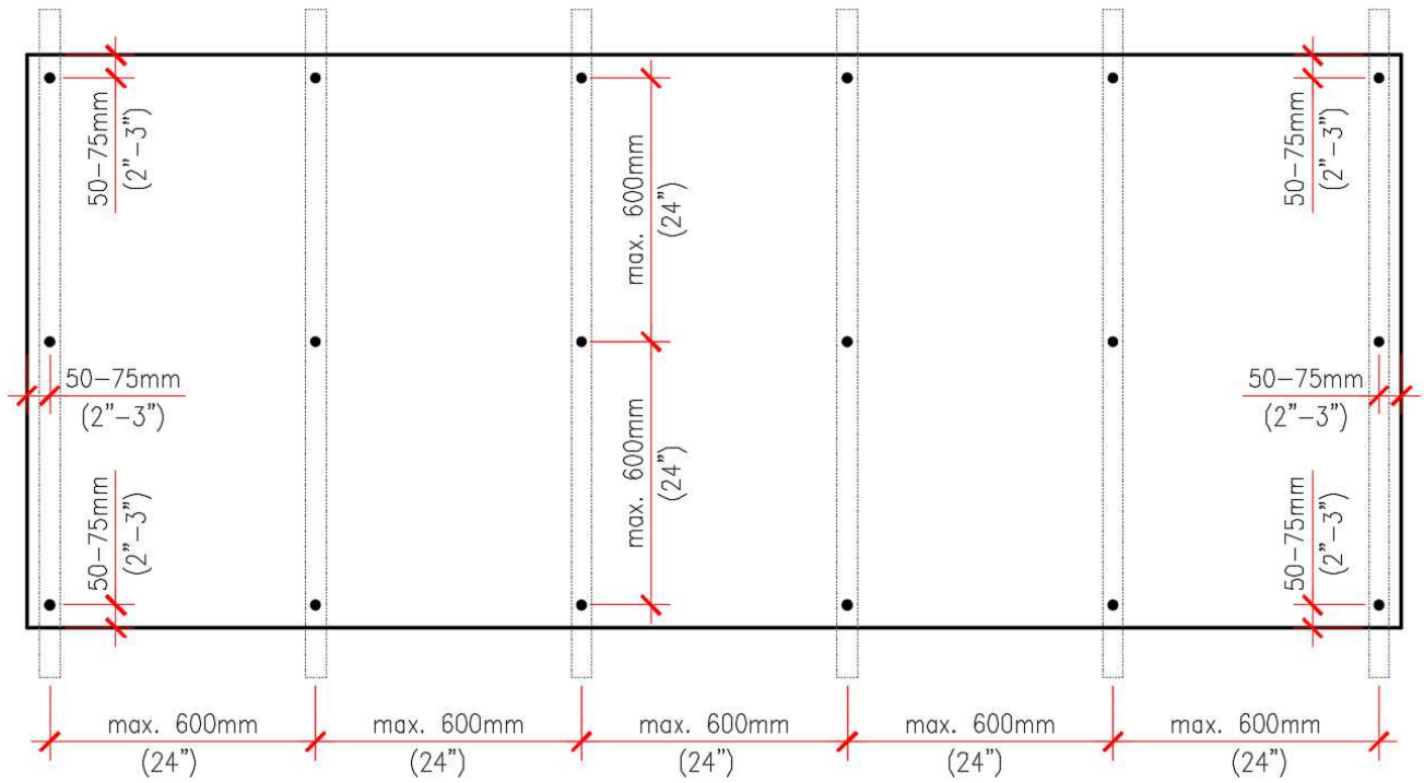
Schéma 4.1 – Emplacement des fixations
