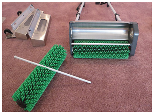
19 Align Bar & Brush and Push until it slides all the Through – DO NOT FORCE Alinee la barra y el cepillo y empuje hasta que se deslice completamente- NO FUERCE
