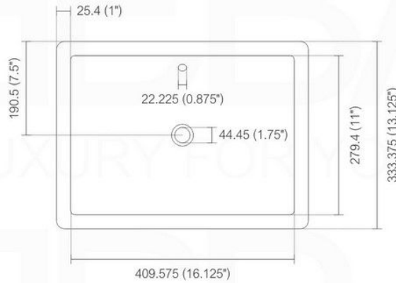
TOP ELEVATION
