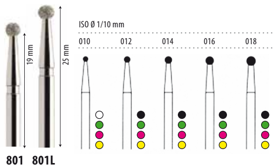
FRESA DE DIAMANTE TIPO BOLA Disponible también en tallo largo
