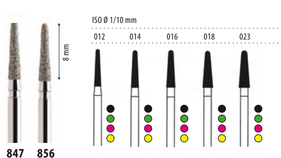
FRESA DE DIAMANTE CONICA PUNTA REDONDEADA / PLANA 8 MM DE PARTE ACTIVA
