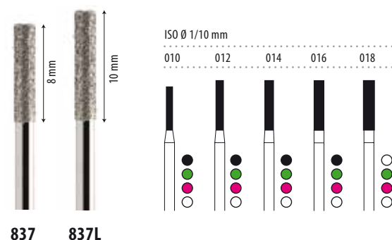
FRESA DE DIAMANTE TIPO CILINDRO CON PUNTA PLANA
