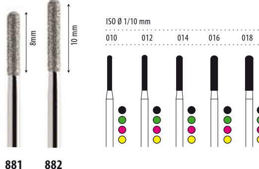
FRESA DE DIAMANTE TIPO CILINDRO CON PUNTA REDONDEADA
