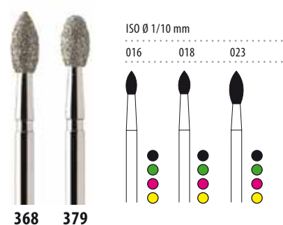
FRESA DE DIAMANTE TIPO BALON DE RUGBY
