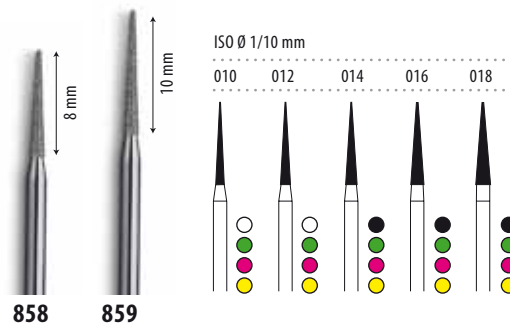
FRESA DE DIAMANTE TIPO LANZA O INTERPROXIMAL
