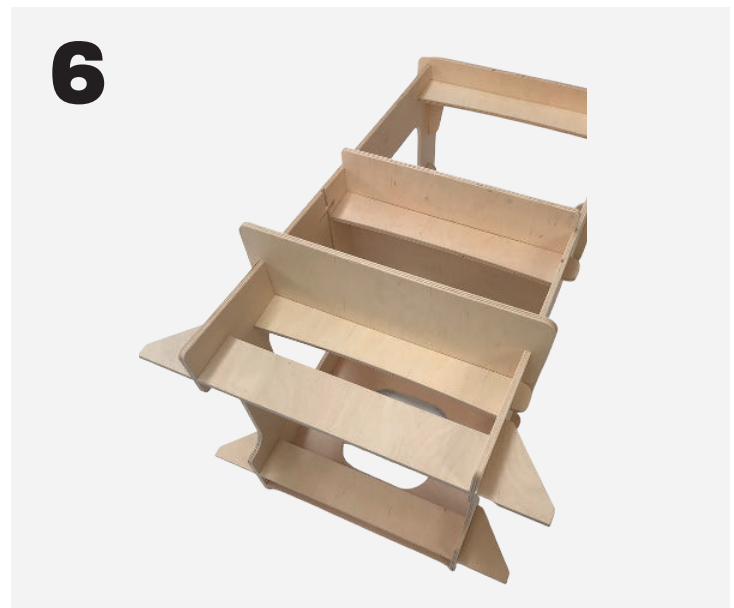
Læg tårnet ned på ryggen og påmonter de 2 fødder (G) på bunden.
