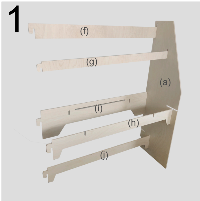
1 Indsæt de 5 store afstiver (f)(g)(h)(i)(j) i 1 side (a)
