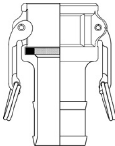
Tipo C Acople Hembra x Vástago para Manguera
