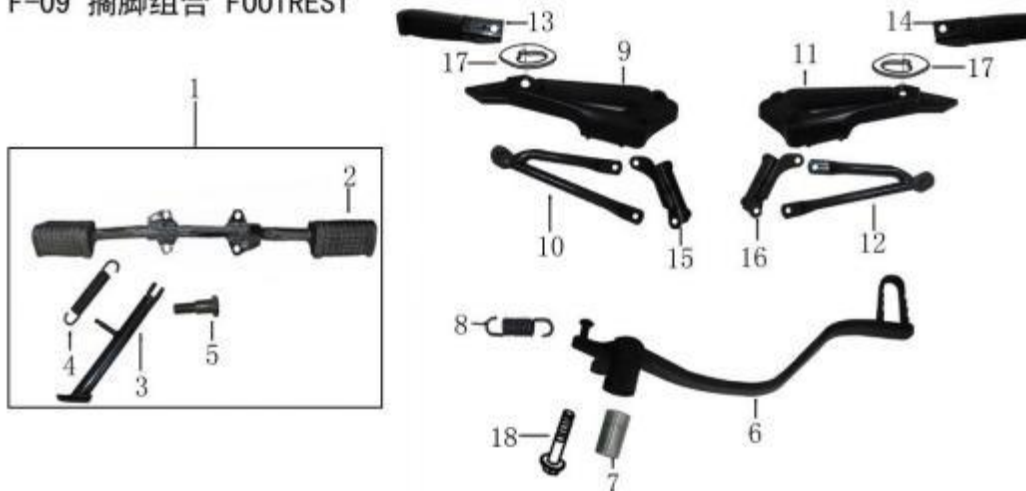
F-09 搁脚组合 FOOTREST
