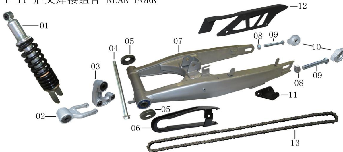
F-11 后叉焊接组合 REAR FORK
