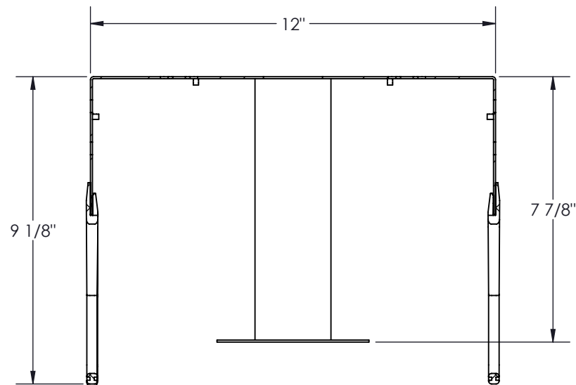
COUPE B-B ÉCHELLE 1 : 4
