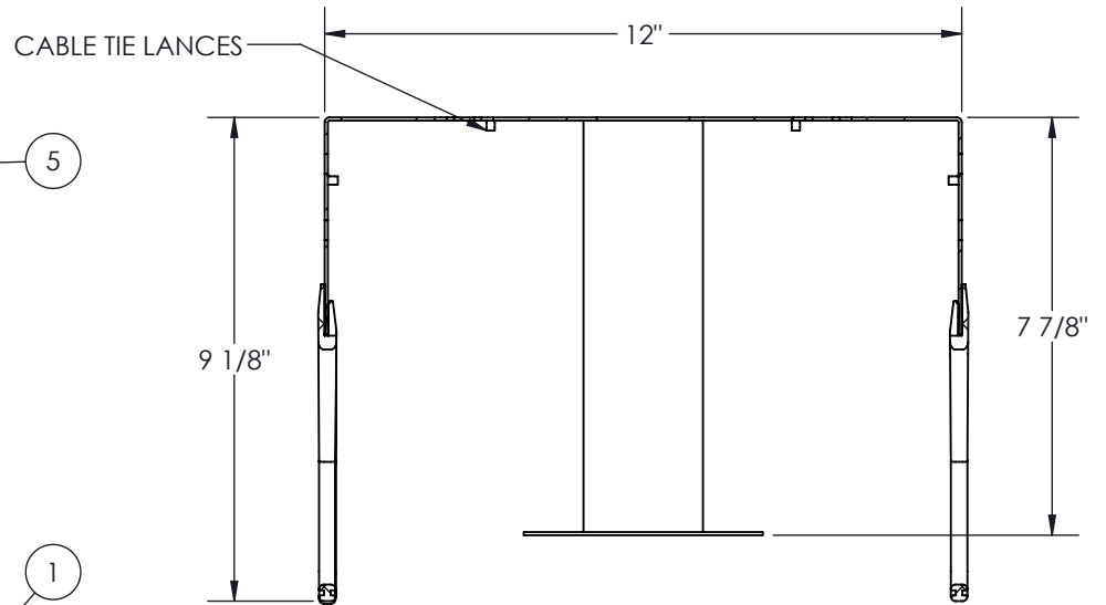
SECTION B-B SCALE 1 : 4
