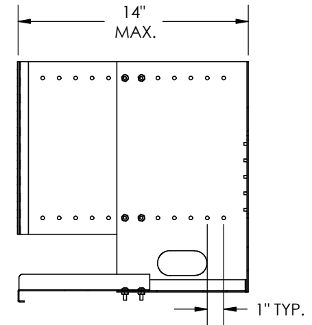
SECTION A-A 14" DEEP
