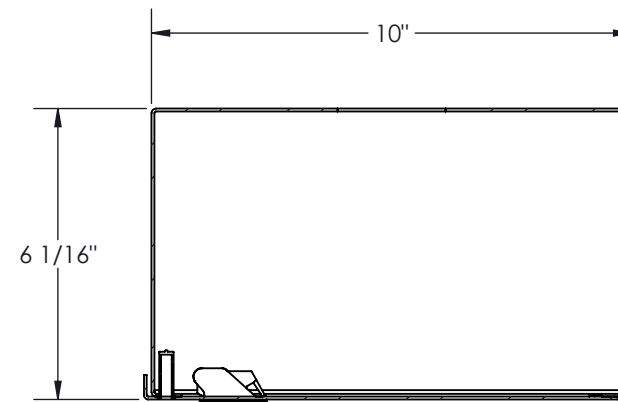
SECTION B-B SCALE 1 : 4
