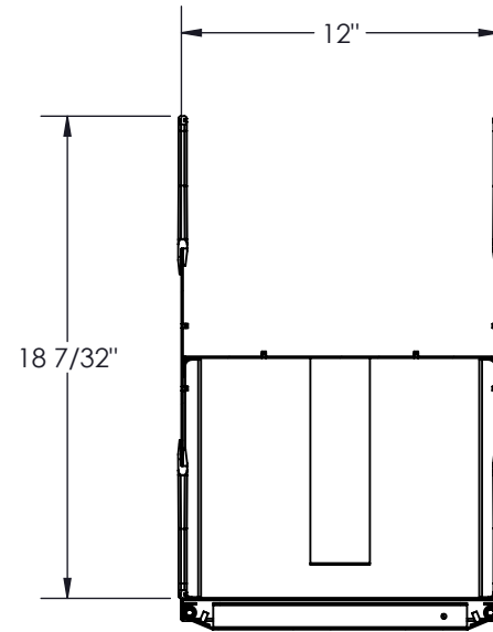
SECTION B-B SCALE 1 : 8
