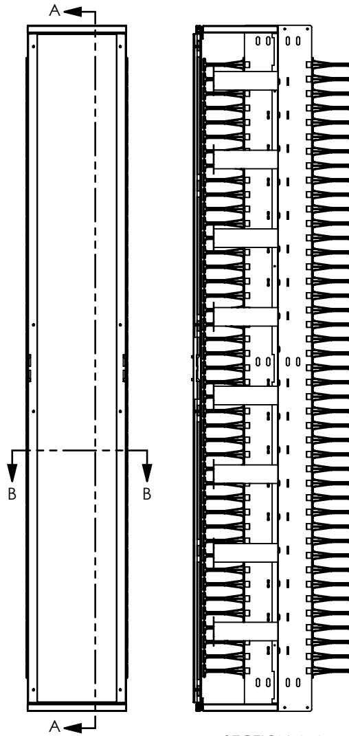
SECTION A-A
