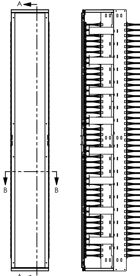
COUPE A-A ECHELLE 1 : 18
