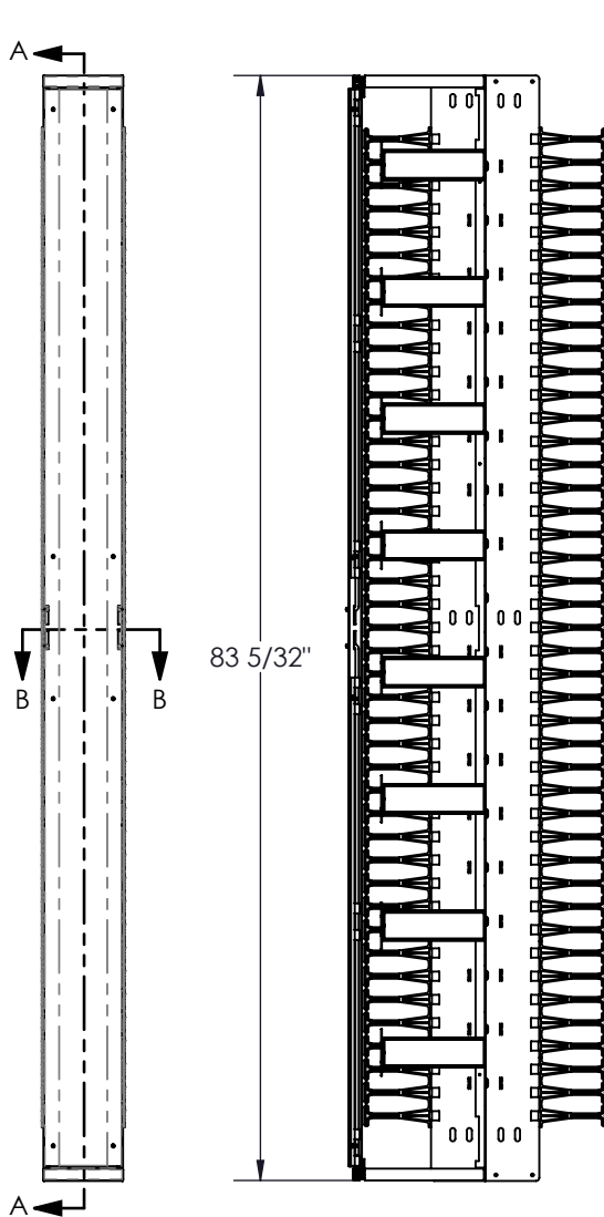
SECTION A-A
