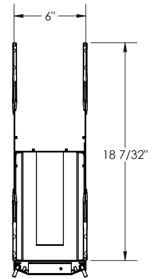
COUPE B-B ECHELLE 1 : 8
