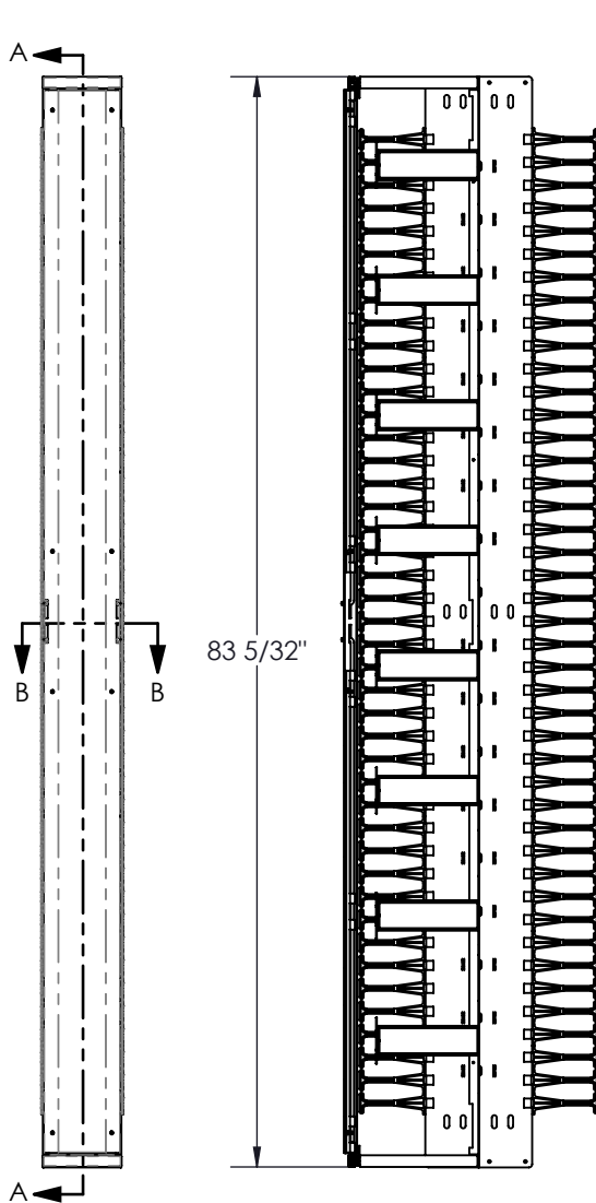
COUPE A-A
