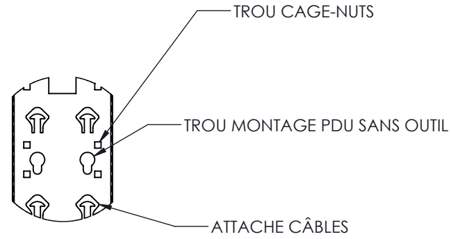
DÉTAIL L ÉCHELLE 1 : 8
